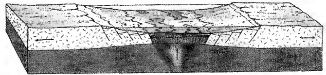
مرحلة تكون بحر طولي ضيق مثل البحر الأحمر
